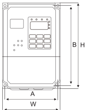
Рис.2.4- Внешний вид и размеры ПЧ ( \leq 22 кВт)
