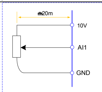
Рис. 3.7- Схема подключения к аналоговому входу ПЧ
