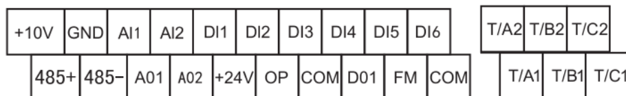
Рис.3.5- Клеммы управления.
