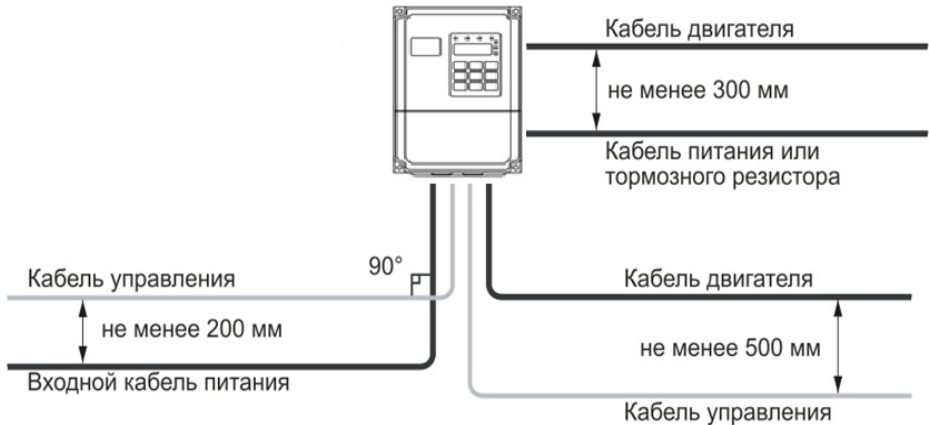
Рис. 3.6- Схема расположения кабелей преобразователя частоты
